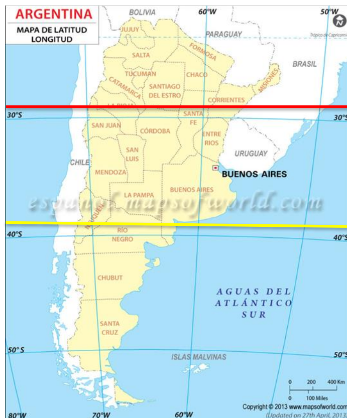
Figura 2. Distribución estimada del GBG en Argentina (paralelos 29 y 39 líneas roja y amarilla, respectivamente)
